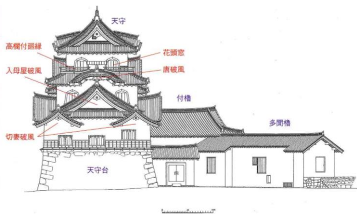
国宝彦根城天守附櫓及び多門櫓 立面図
