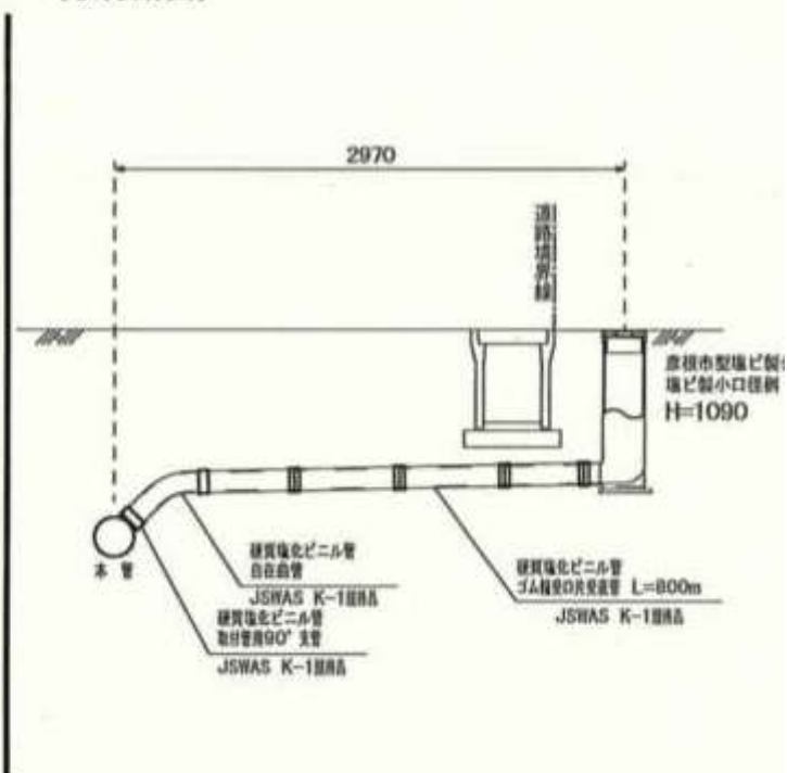
(取付断面)
