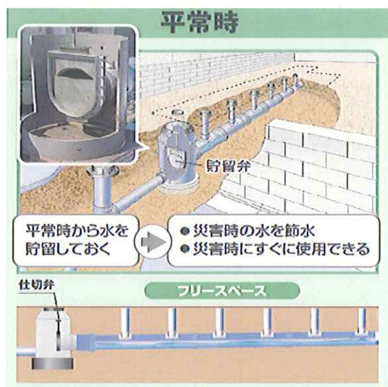
資料2 災害用マンホールトイレ下部構造図 (イメージ図)
