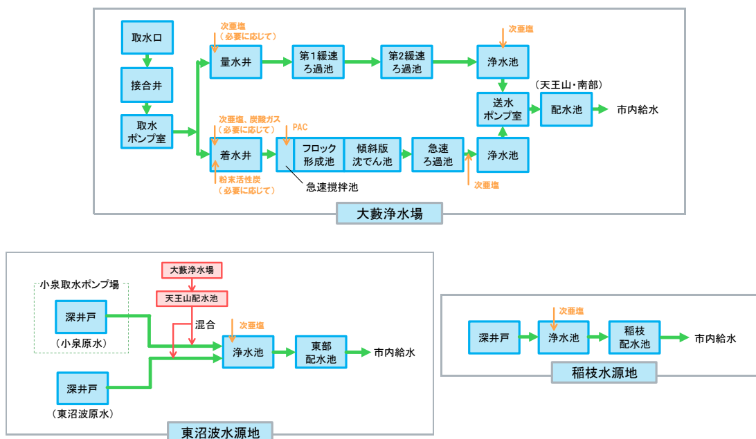
浄水フロー
