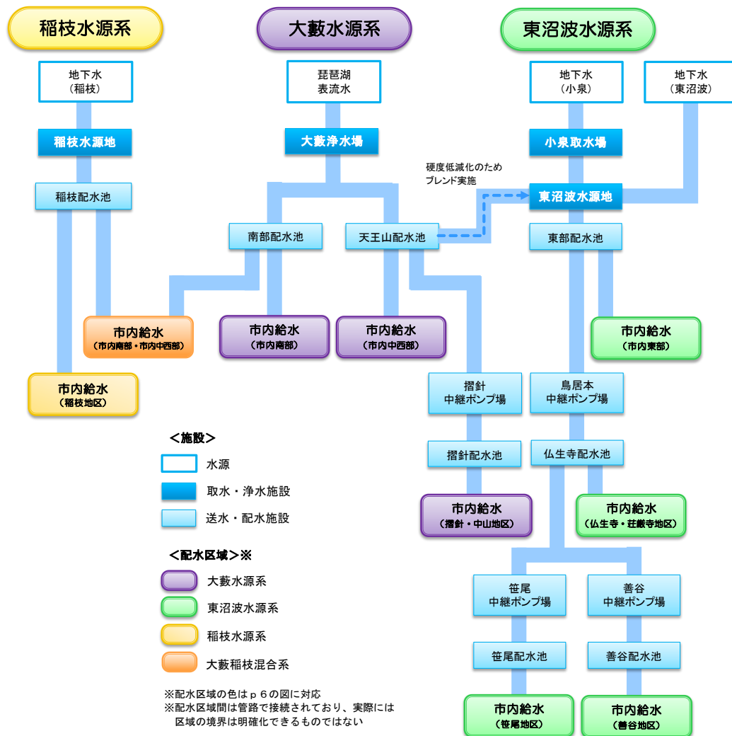
配水フロー
