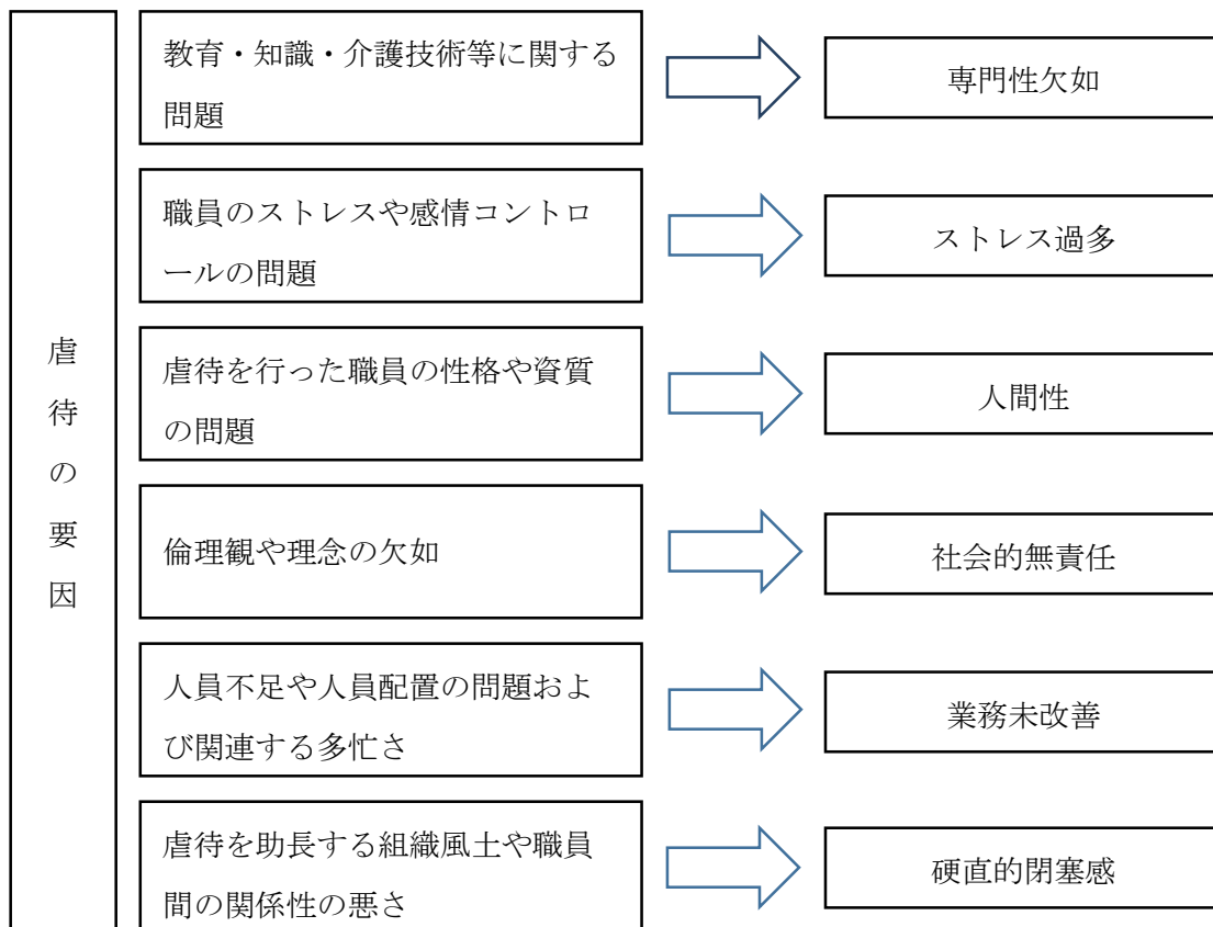
図 4.1 虐待の要因
