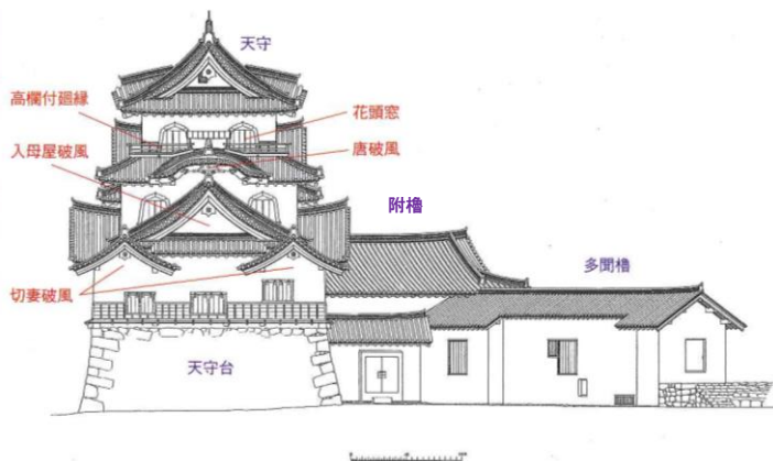
国宝彦根城天守附櫓及び多聞櫓 立面図
