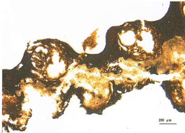
2号横带上層突帯部の横断面 ※バーの長さは200μm (0.2mm)
