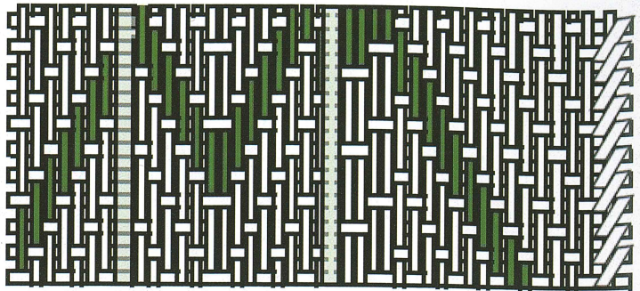
1号横带上層外面の組織模式図
