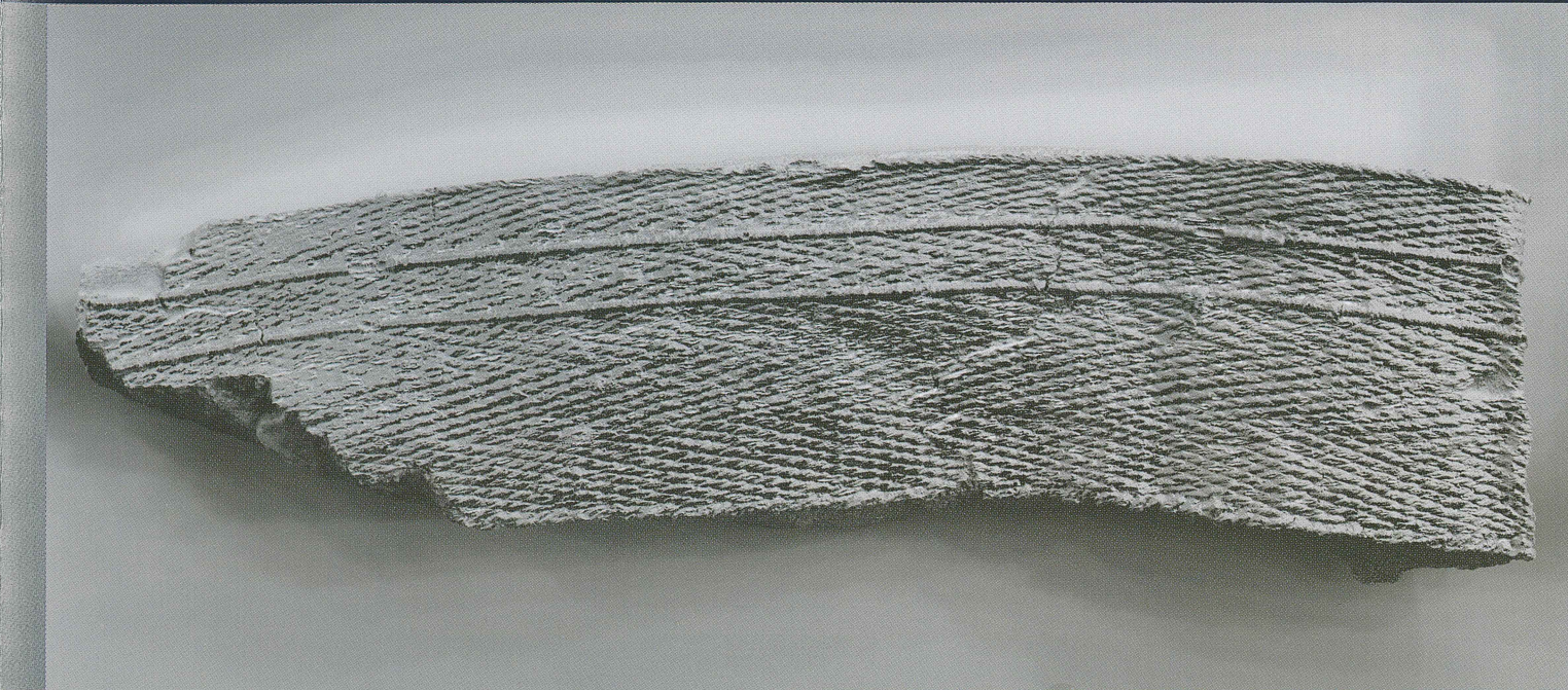
2号横带上層突帯部の縦断面 撮影 公益財団法人元興寺文化財研究所
