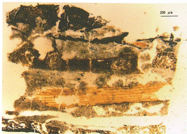
2号横带上層突帯部の縦断面 撮影 公益財団法人元興寺文化財研究所
