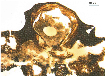
2号横带上層突帯部の横断面
