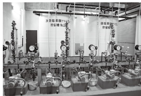
▲薬品注入設備
