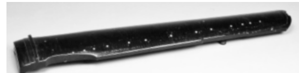
▲写真2: 七絃琴
