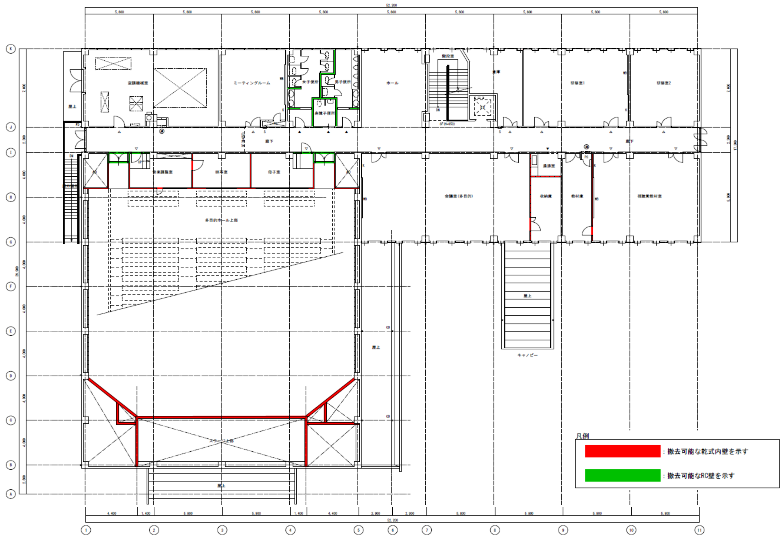
図 8 撤去可能な壁の図示(2 階)
